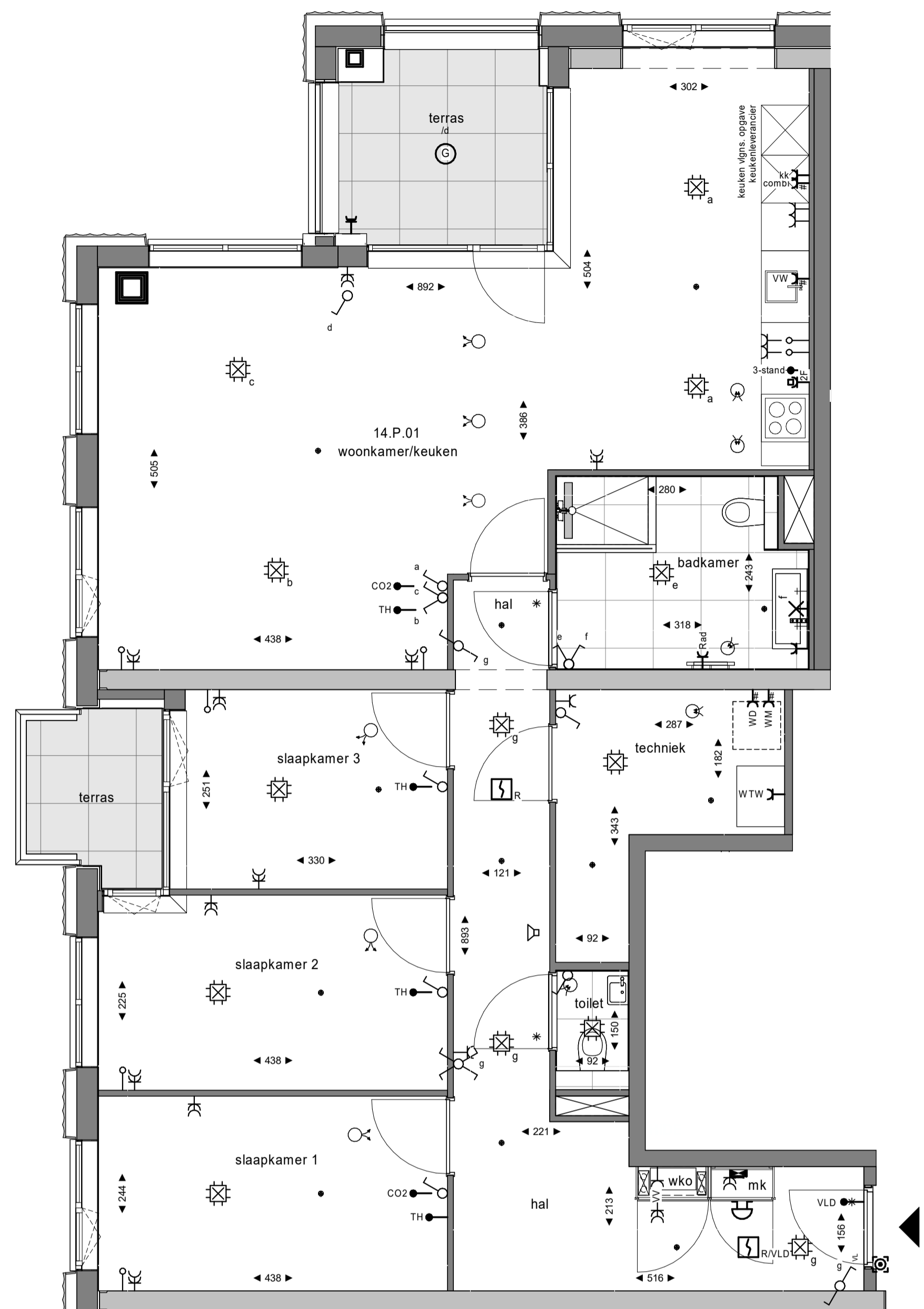
plattegrond 1 : 50 14e verdieping
