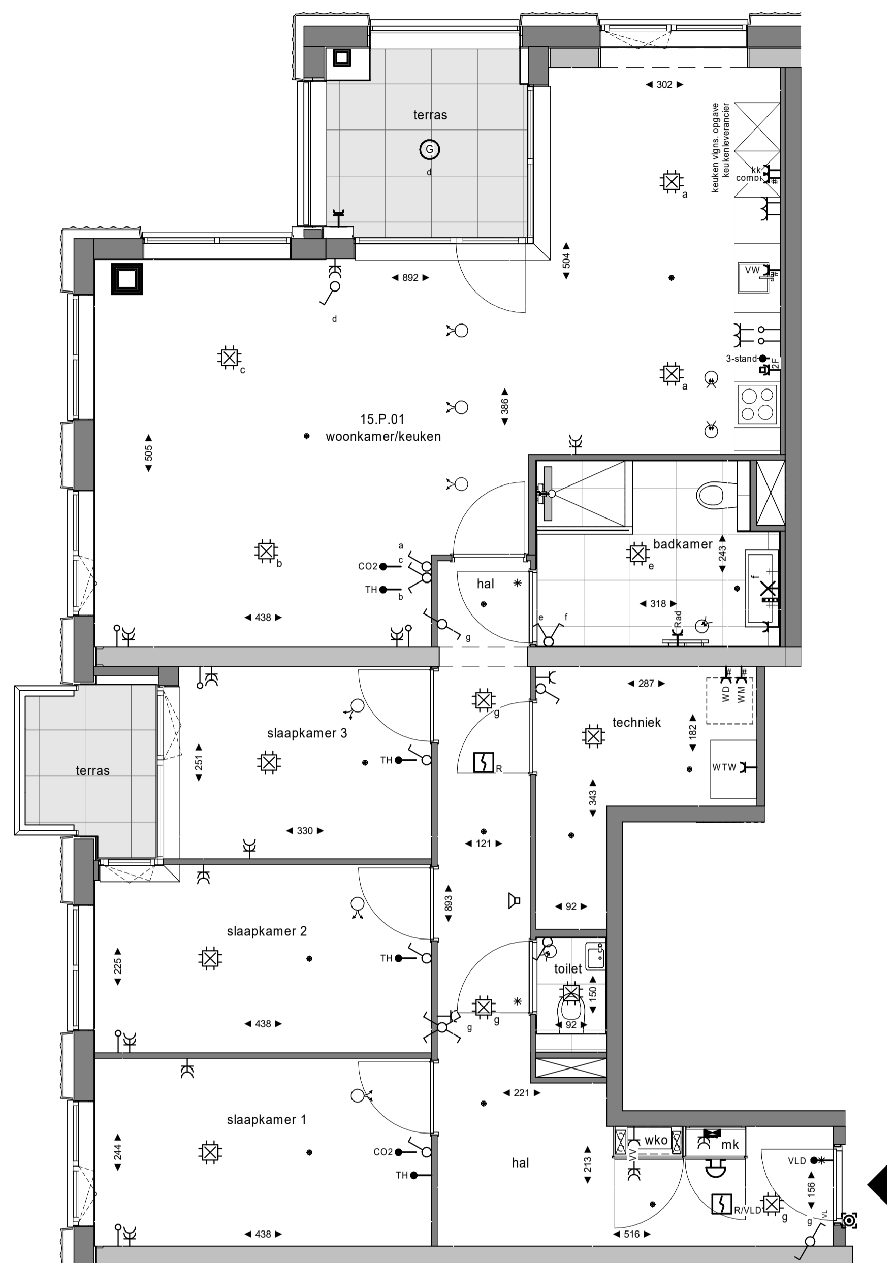
plattegrond 1 : 50 15e verdieping
