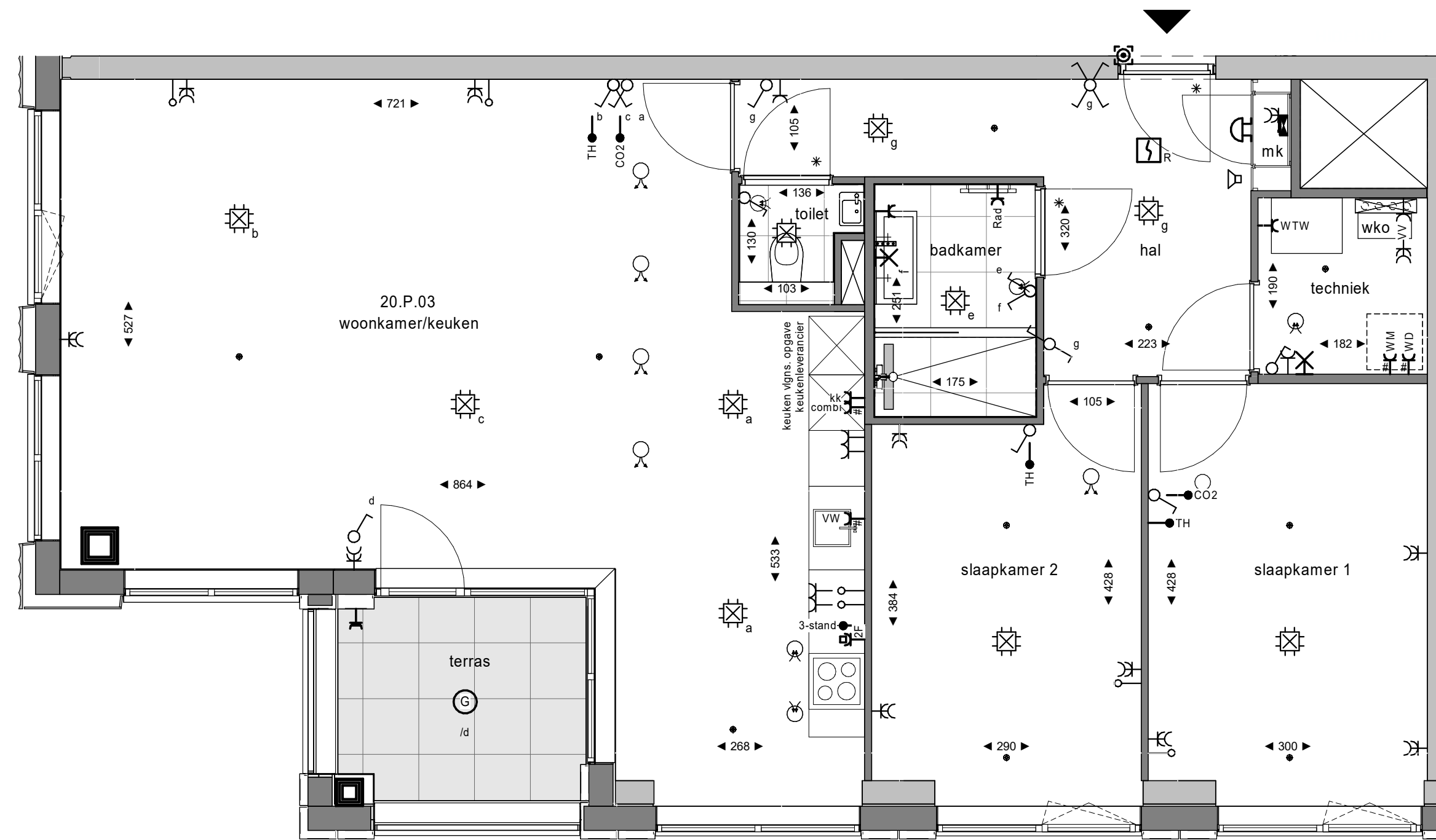
plattegrond 1 : 50 20e verdieping
