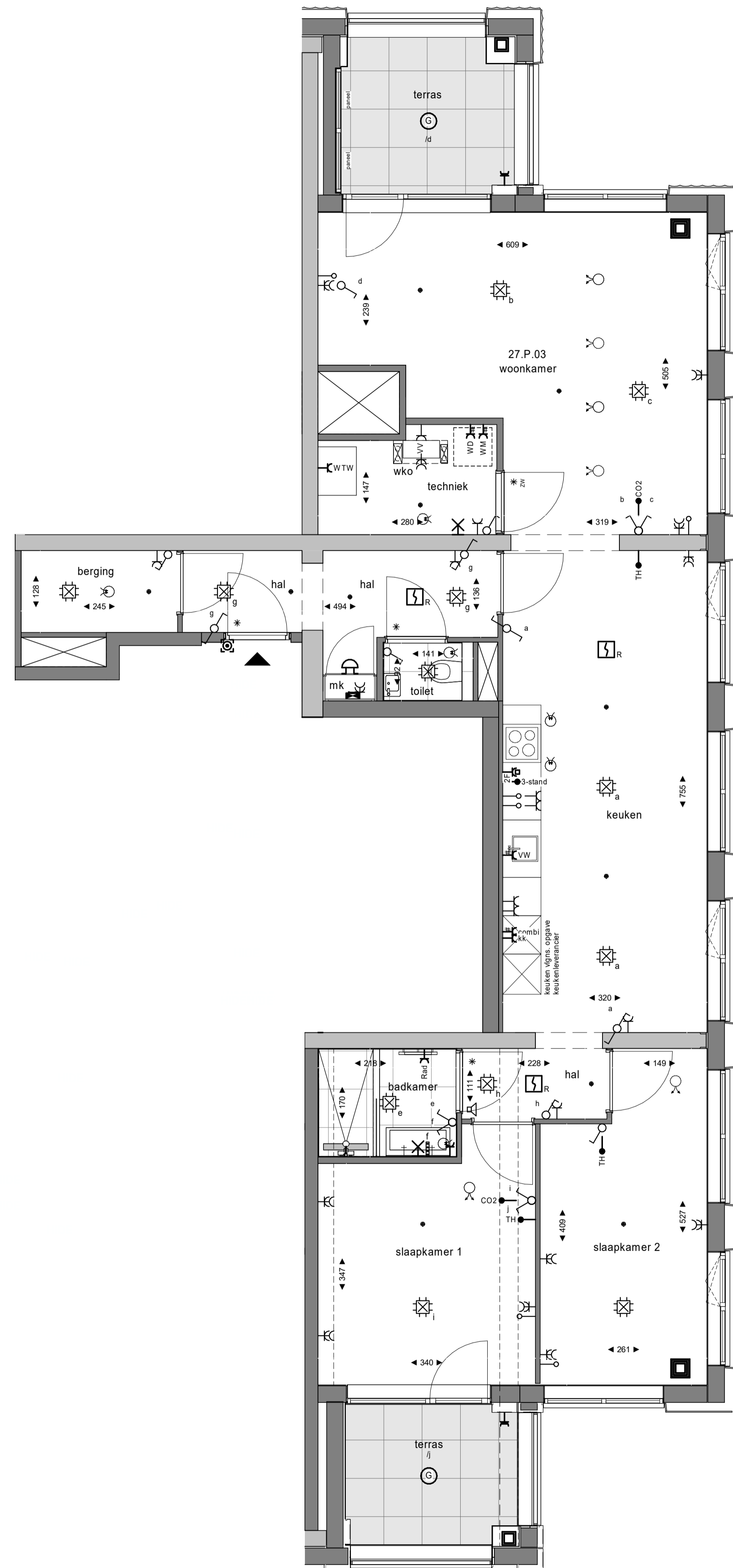
plattegrond 1 : 50 27e verdieping
